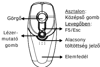
Felülnézet
